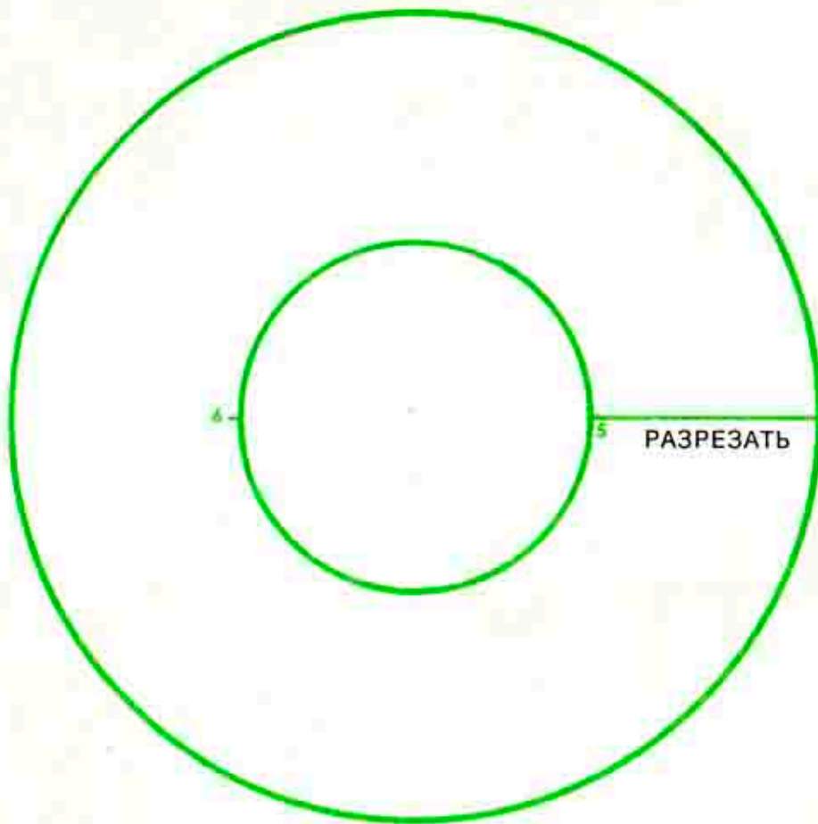
ДЕТАЛЬ ВОЛАНА ПЛАТЬЯ В НАТУРАЛЬНУЮ ВЕЛИЧИНУ
